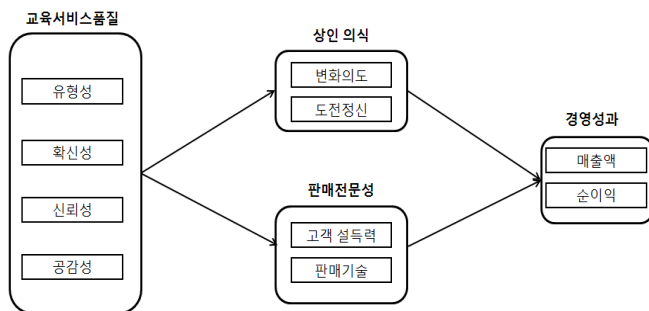
<그림 2> 연구모형
