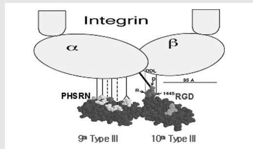
그림 4. Fibronectin III형의 10번째와 9번째 도메인의 RGD와 PHSRN 아미노산이 integrin과 결합하고 있는 모습.
