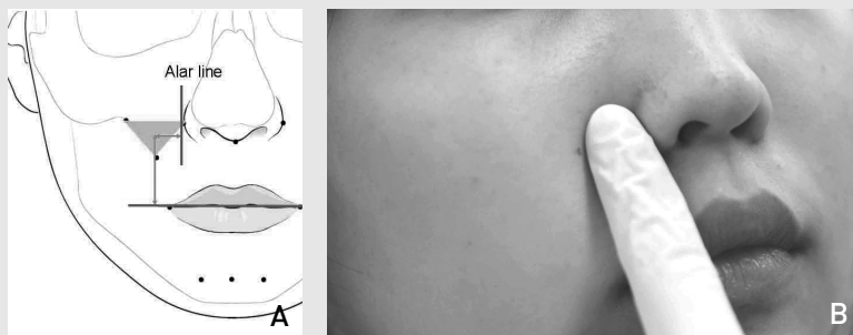
그림 3. 시체 해부 연구를 통해 입꼬리를 당기는 근육을 가장 효과적으로 이완시키는 주사점, alar point에서 1cm 측방에 위치한다(A). 실제 환자에서 주사하는 모습(B).
