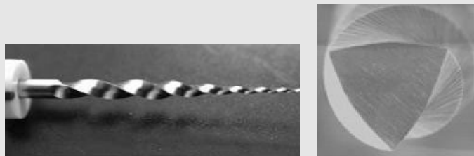
A: 측면날의 형태가 날로 구성됨-ProTaper B: 날의 형태를 가진 단면형태
