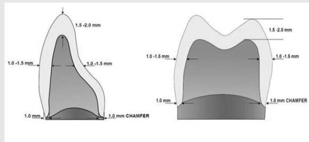
그림 15. CAD/CAM 밀링 시 오류를 최소화 할 수 있는 치아 삭제 형태
