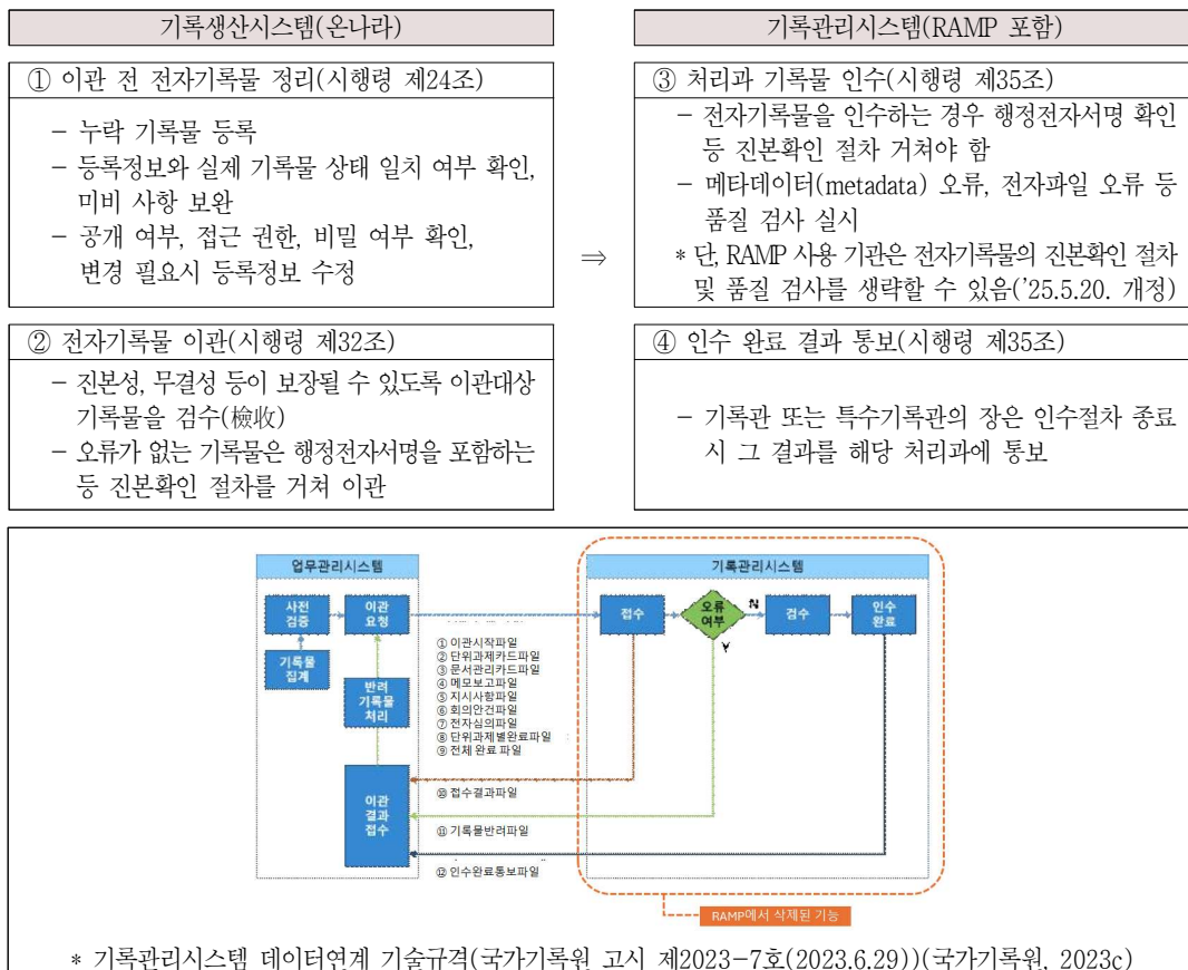
<그림 3> 「공공기록물법 시행령」상 처리과 전자기록물의 기록관리시스템 인수 절차와 내용
