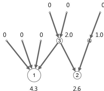
<그림 4> 그림 1의 인용 네트워크에서 논문별 CCI를 측정한 결과
