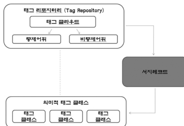
<그림 7> 태그 리포지터리의 구조
