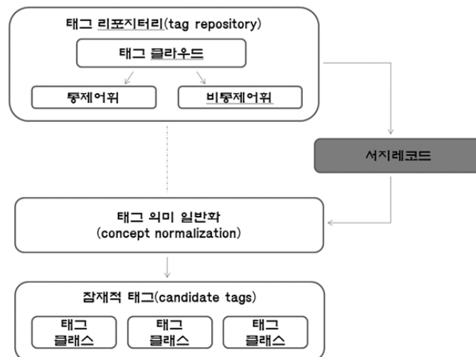
〈그림 8〉 태그의 의미 일반화 과정
