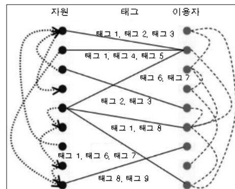
〈그림 2〉 태깅시스템의 모델 (출처: 이성숙, 정서영 2009)
