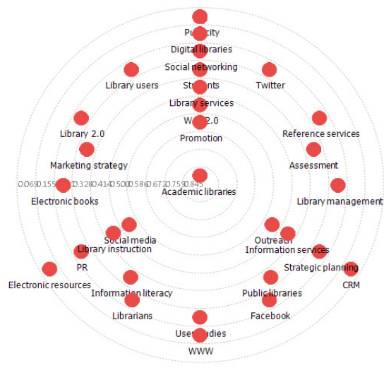
〈그림 9〉 국외 논문 키워드의 연결 중심성 Concentric
